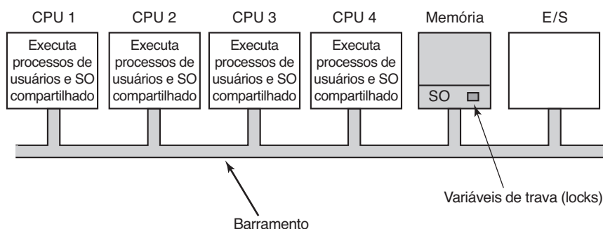
FIGURA 8.9 O modelo de multiprocessadores simétrico (SMP).
