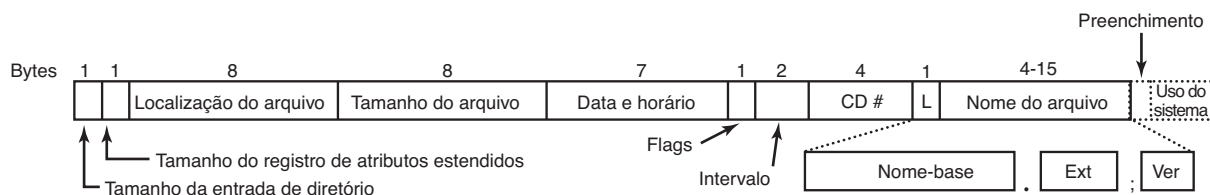
FIGURA 4.35 A entrada de diretório do ISO 9660.
